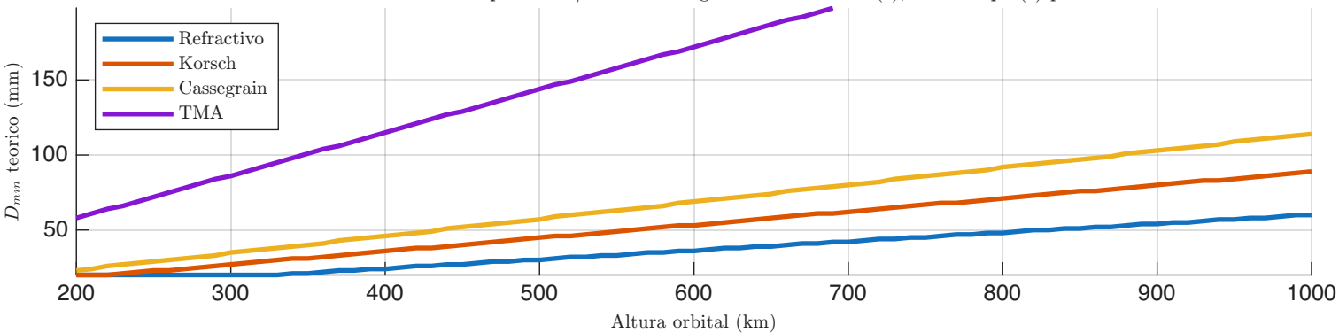
Detector 3: mínimo teórico por MTF/SNR - Configuración: 2 satélite(s), 1 telescopio(s) por satélite
